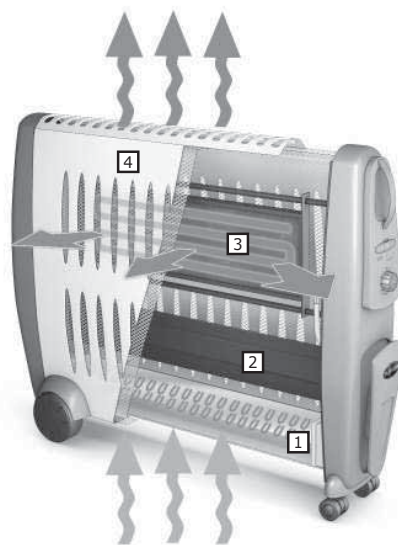
Fig. 13 : Fonctionnement du radiateur CERAM DUO
