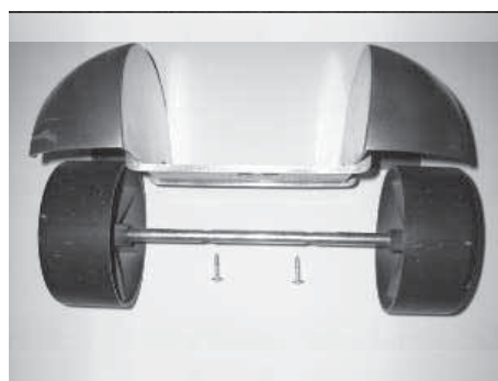
Fig. 5 : Ensemble roues arrières D
