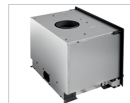
Carénage complet : dessus prépercé pour 4 buses de distribution d'air chaud. (NÉO 76, 76 16/9ème et 67)
